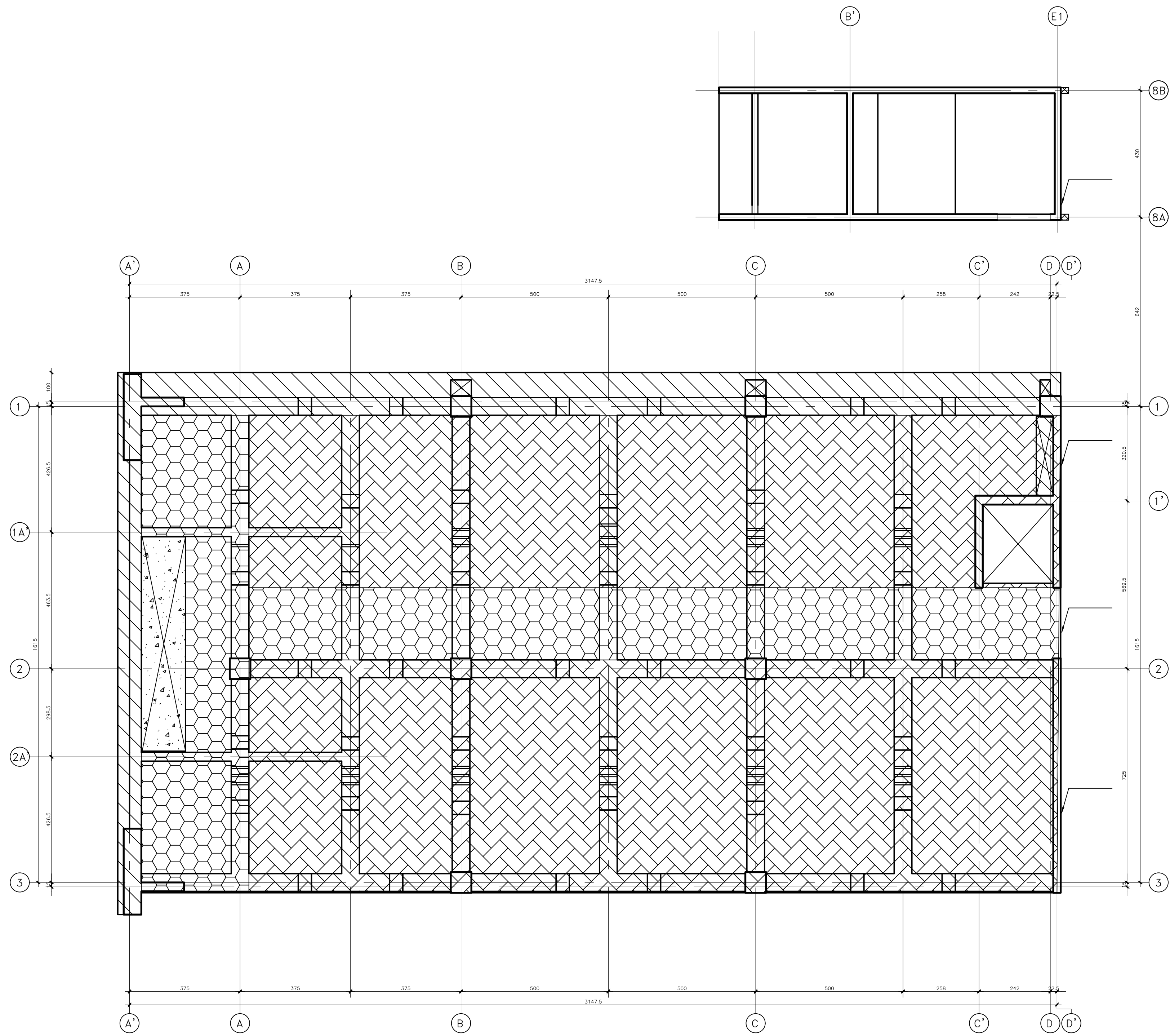
PLANTA CARGAS CIELO 1°SUBTERRANEO a CIELO PISO 3°
