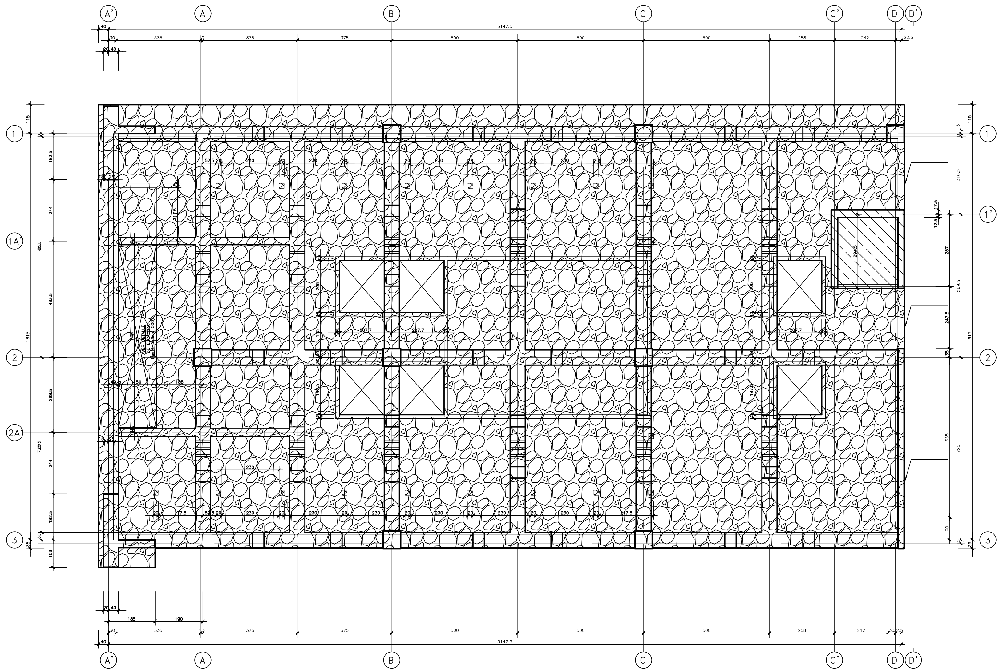
PLANTA CARGAS CIELO PISO 4°
